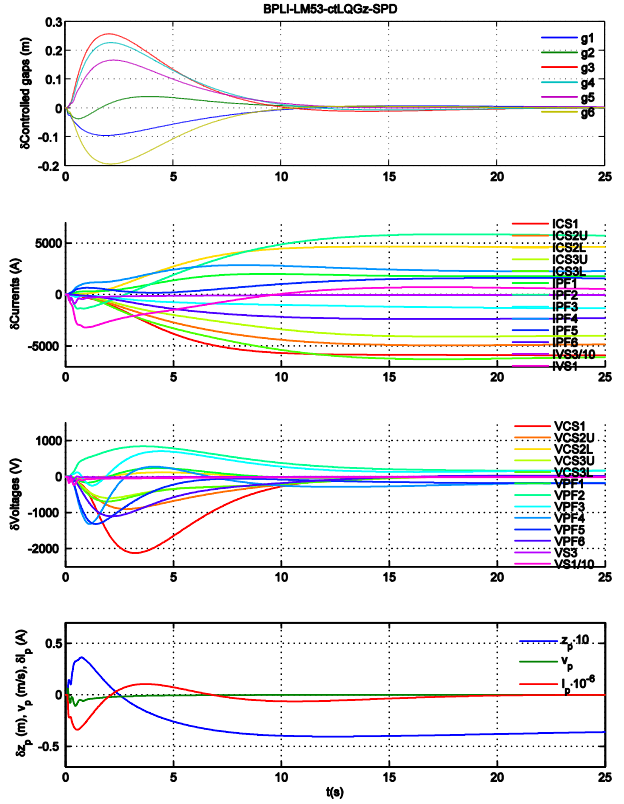
Fig. 4. BPLI simulation: ctLQGz-SPD, model LM53.
