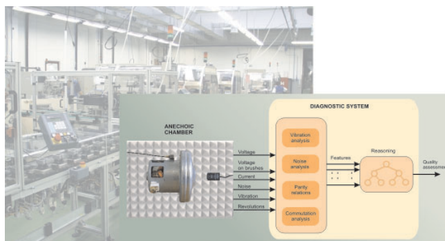
Slika 2. Sistem za končno kontrolo kvalitete elektromotorjev
